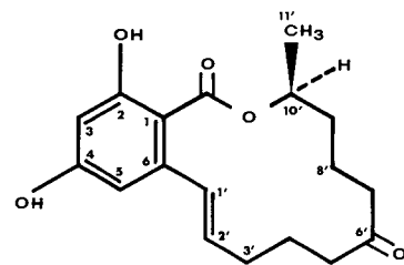
Zearalenone
