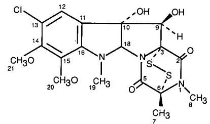
Sporidesmin
